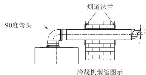
冷凝机烟管图示
