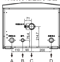
冷凝机水路连接示意图
