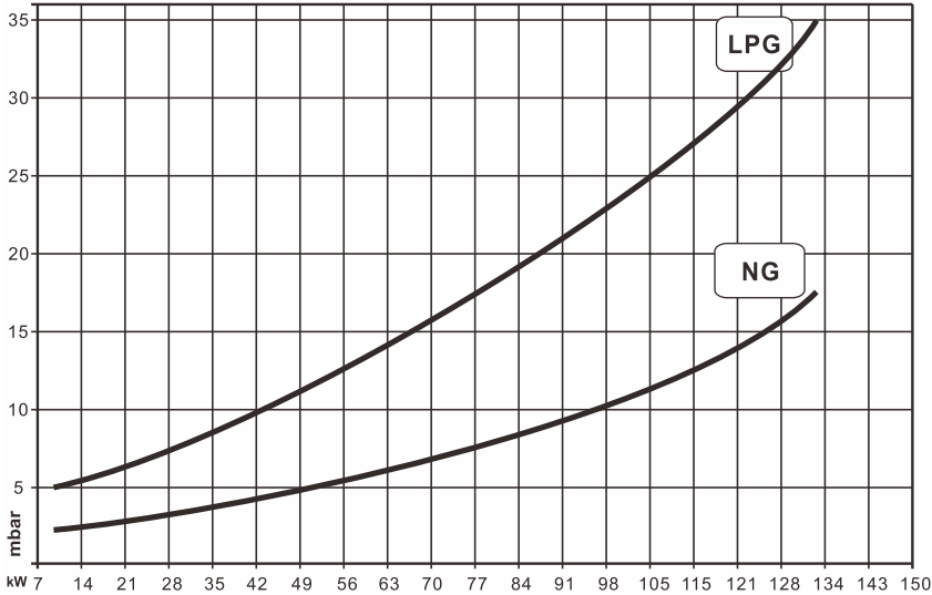
压力-功率曲线图
