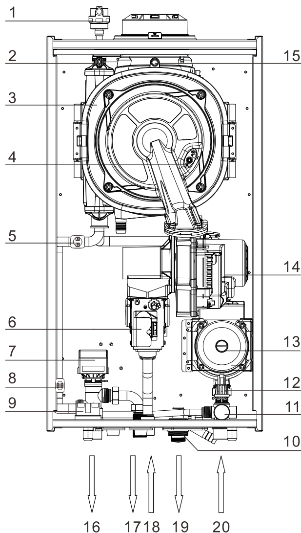
冷凝机结构示意图
