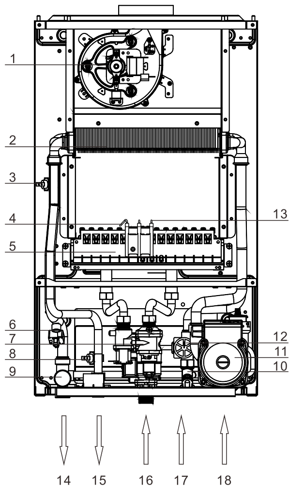
M系列分段机型结构示意图
