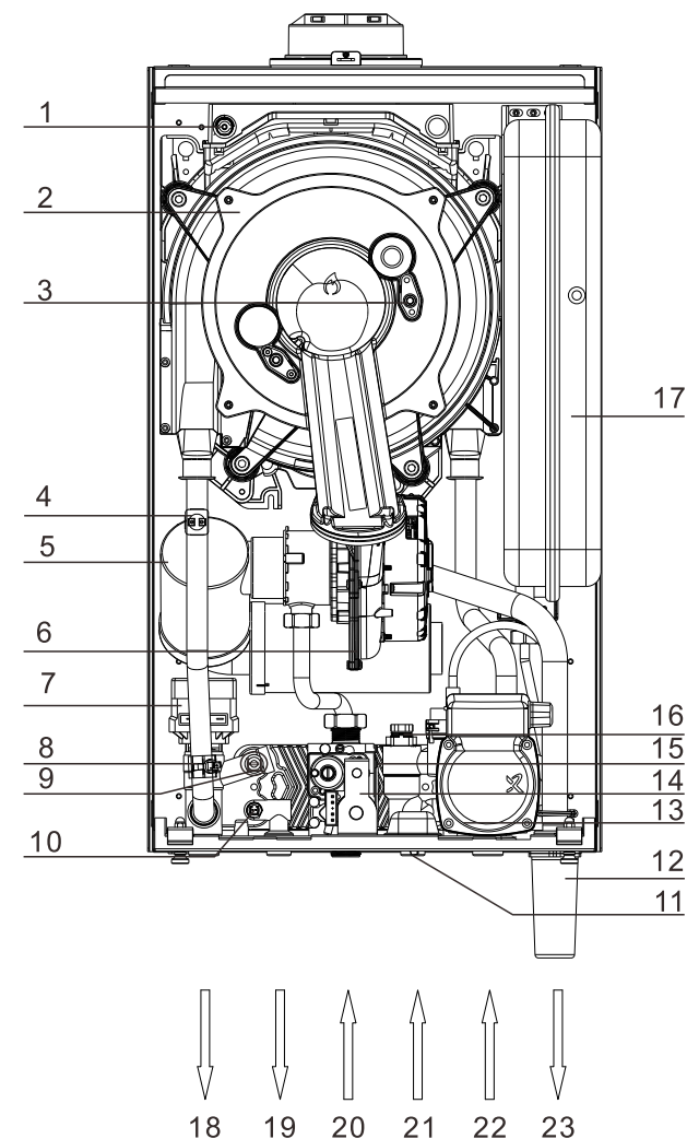
W1系列冷凝机结构示意图
