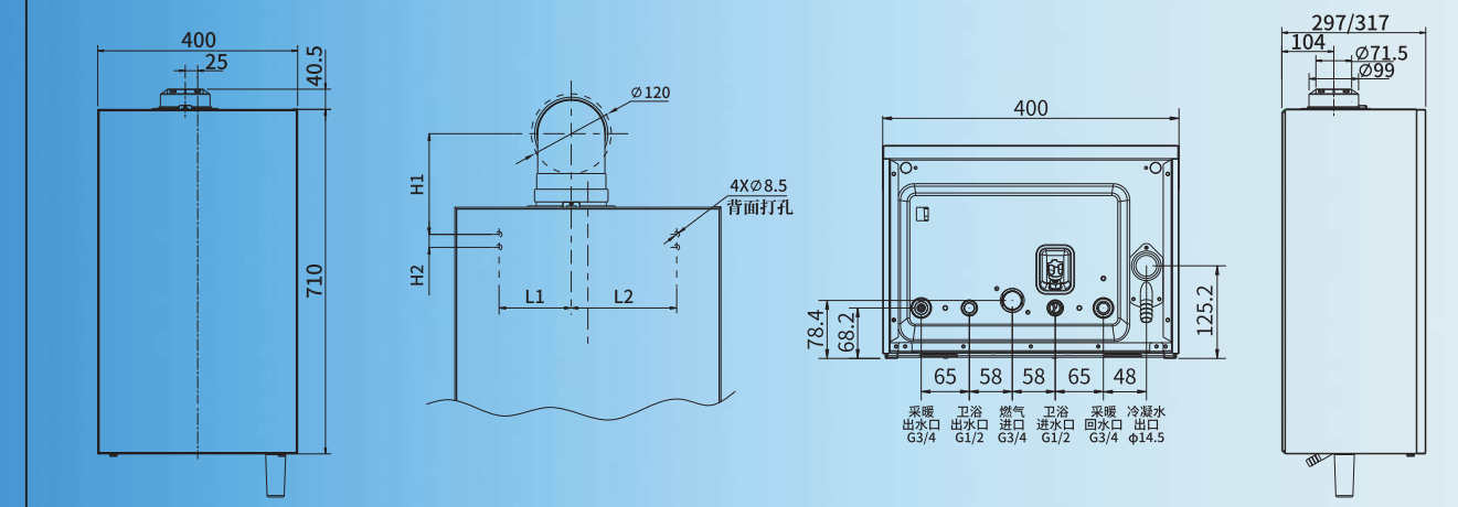
W1系列 产品尺寸及水路连接示意图
